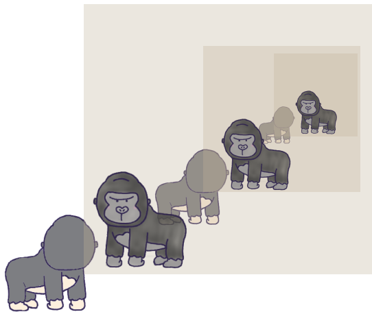
合わせ鏡に映る無限ゴリラ
