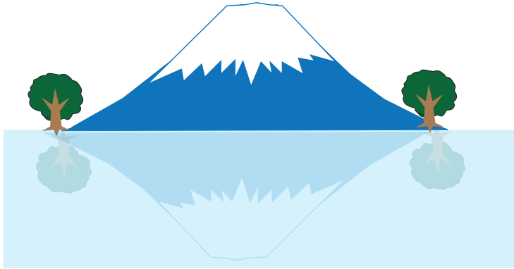
湖に映る富士山
