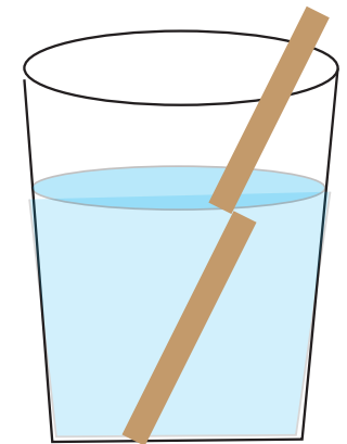
水のはいったコップに 棒をいれるとずれて見える
