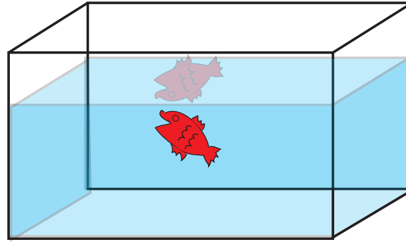
水面に映って見える魚
