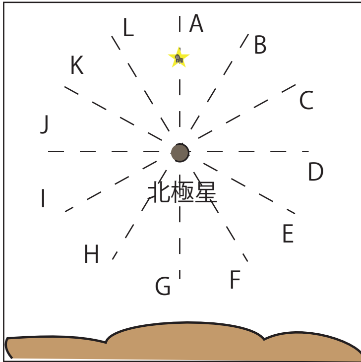
北の空の星の動き
