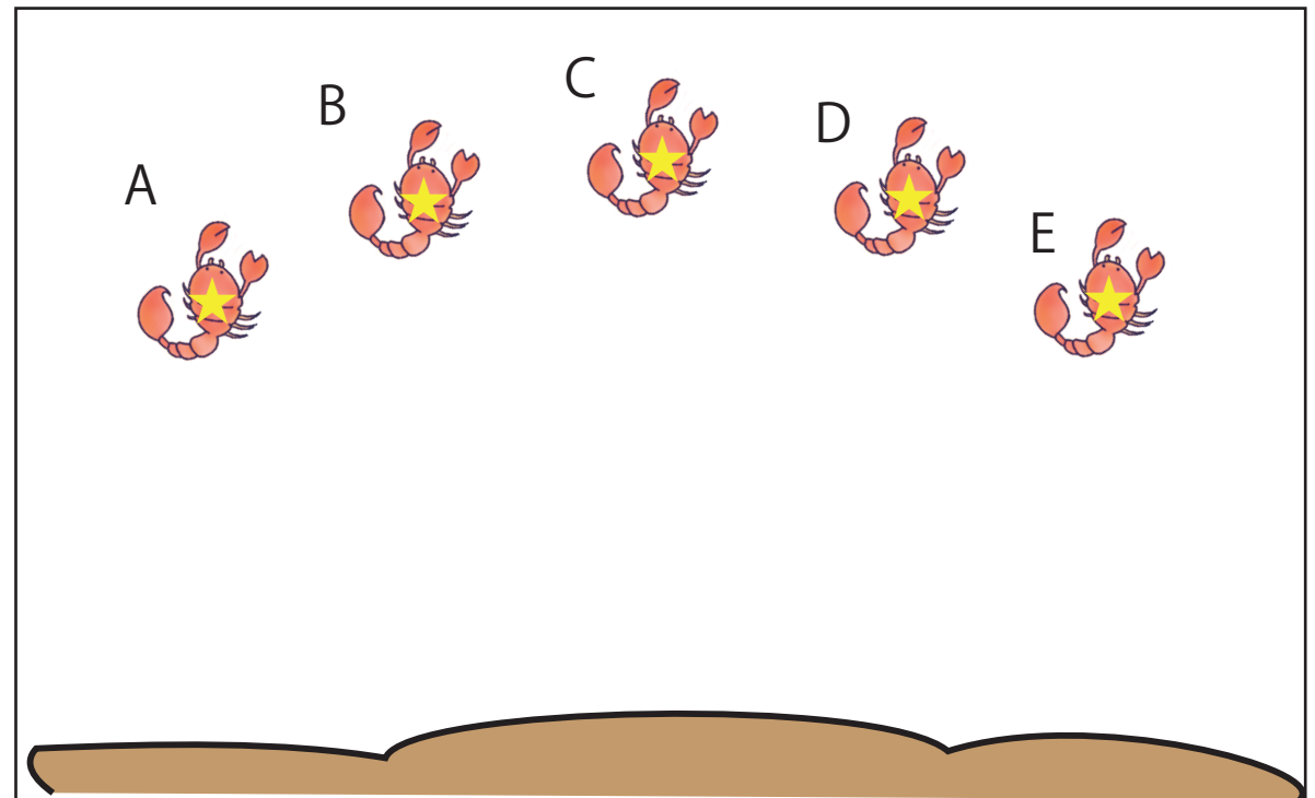
南の空の星の動き
