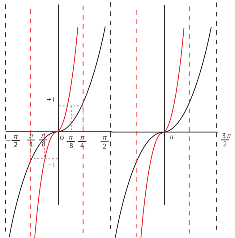
y = \tan(\theta - P) のグラフ
