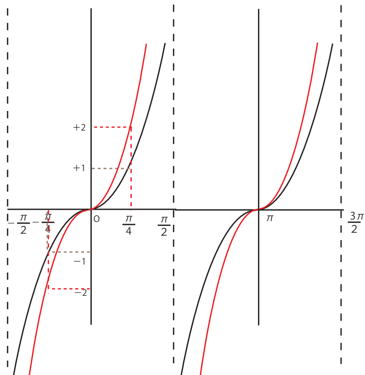
y = 2 \tan \theta のグラフ
