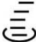
噴火口
